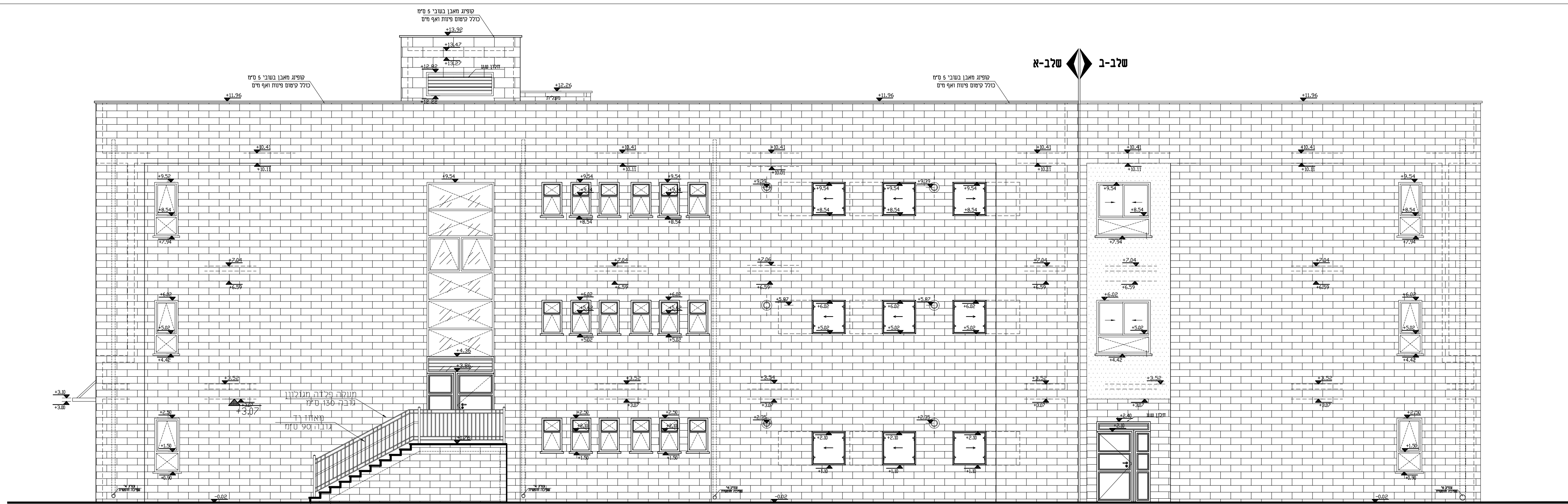
צוית צפונית קו"מ 1:100
